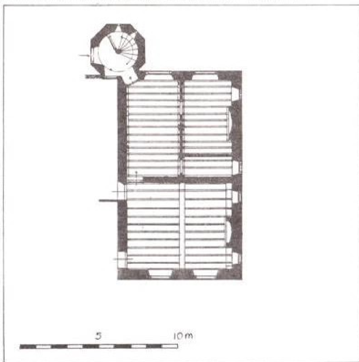
Afb. 4 Plattegrond gelijkvloers. Tekening van W. Scheepens, 1907.
