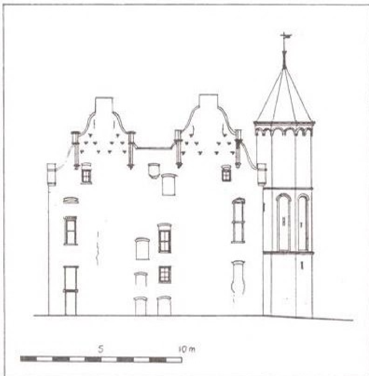
Afb. 2 Zuidgevel van de Loowaard. Tekening van W. Scheepens, 1907.
