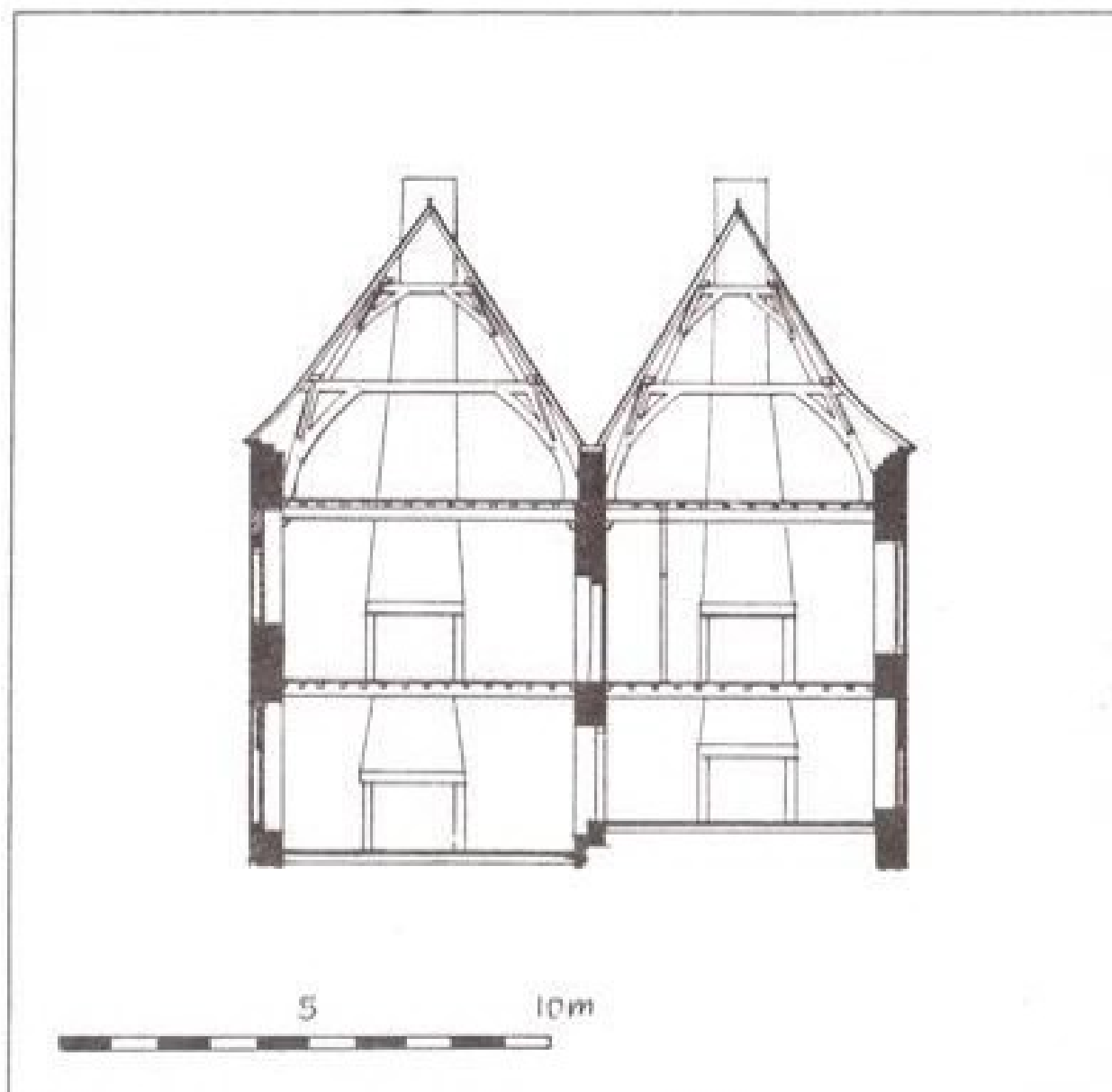
Afb. 5 Doorsnede oost-west. Tekening van W. Scheepens, 1907.
