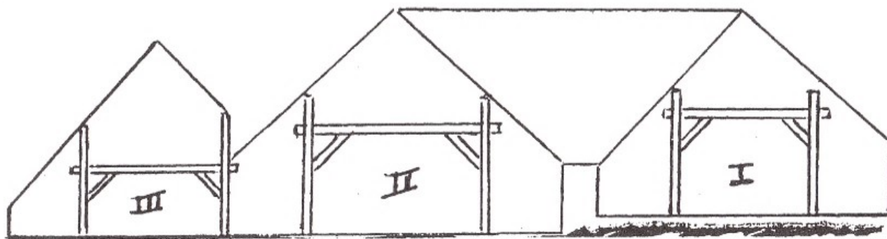
Schematische dwarsdoorsnede van Husselarijstraat 7, gezien naar de achterzijde.
