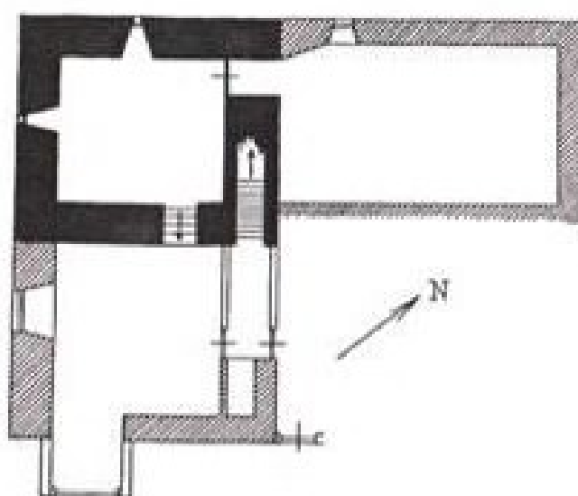
Afb. 2 De begane grond met het oudste deel, de donjon, op de westhoek (ontleend aan het blad 'Cobouw').
